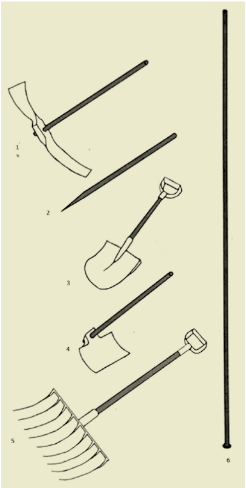
Eines de carboner: 1 pic, 2 donafums, 3 pala, 4 magall, 5 forquilla, 6 burja.
